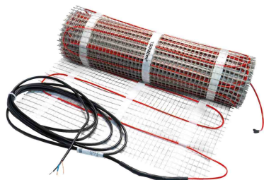
InfraFloor© Fliesenheizung F150A 5m 2 Beispielfoto
