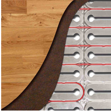
InfraFloor® Parkettheizung P100 15m 2 Beispielfoto
