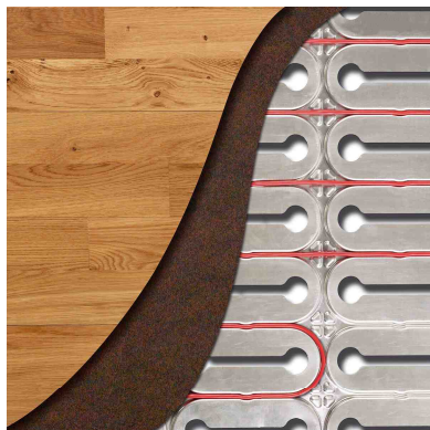
InfraFloor® Parkettheizung P100 16m 2 Beispielfoto
