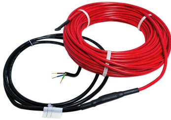
Heizkabel Indoor 52m 230V 18W/m Beispielfoto
